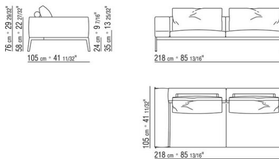
COD. 014C33
