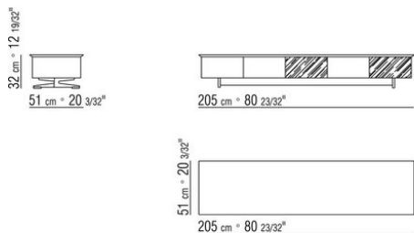
COD. 014X81
